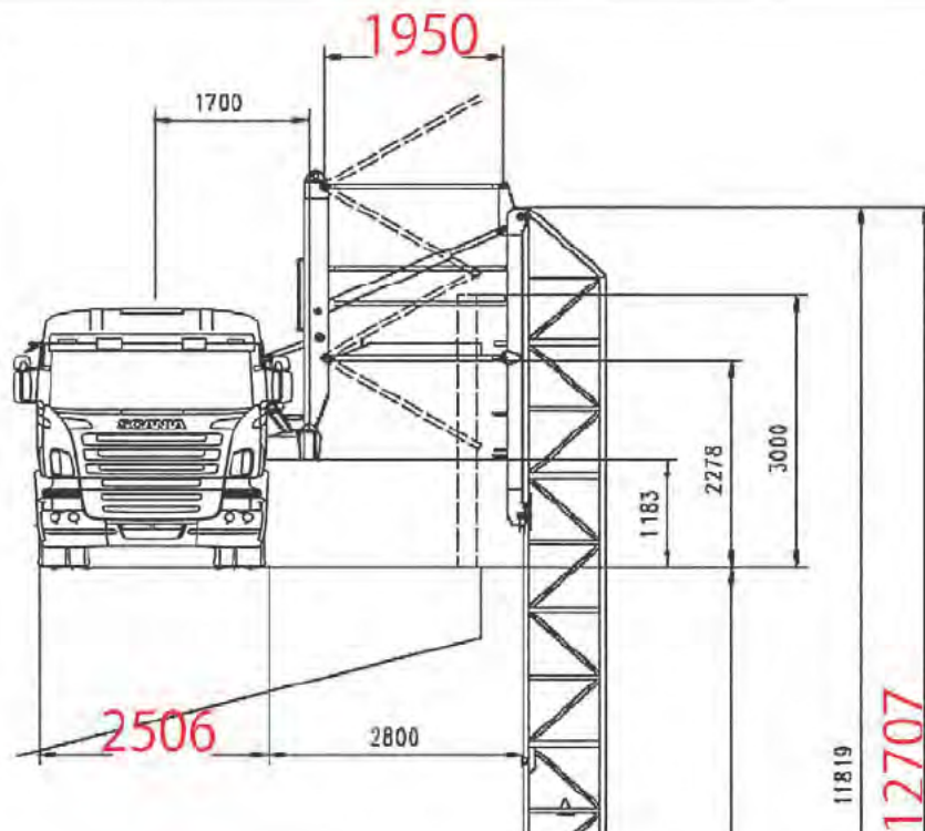
【走行時寸法図】
