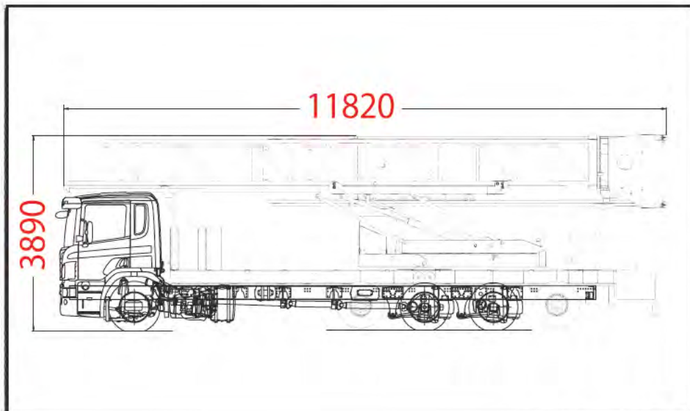
【走行時寸法図】
