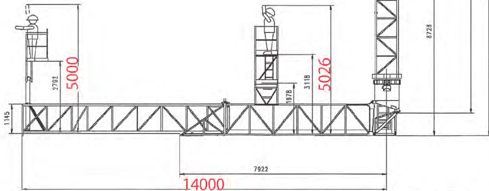
【点検時寸法図】
